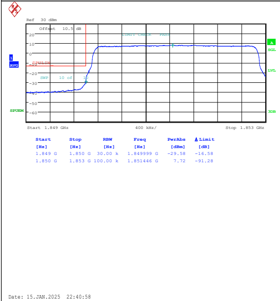
Band2-3MHz-QPSK-18615-15RB#0-PASS
