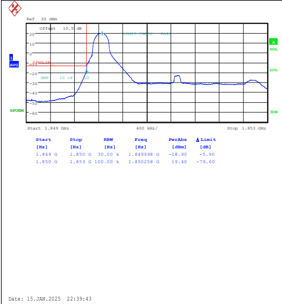
Band2-3MHz-QPSK-18615-1RB#0-PASS
