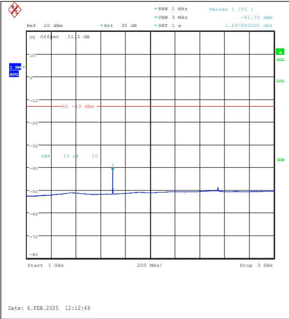
Band26(824-849)-10MHz-QPSK-26990-1RB#49-1 000~3000-PASS
