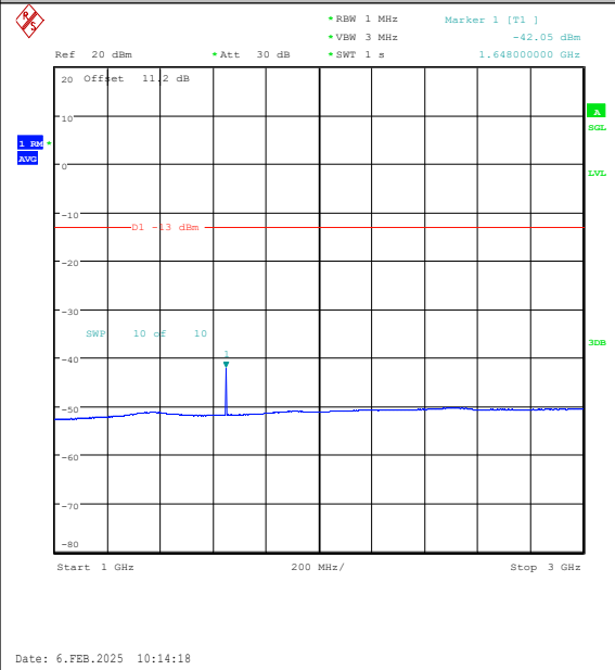
Band26(824-849)-3MHz-QPSK-26805-1RB#0-100 0~3000-PASS
