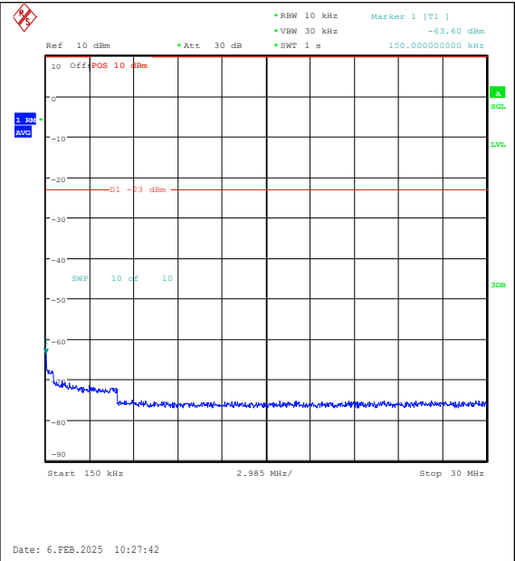
Band26(824-849)-3MHz-QPSK-26915-15RB#0-0. 15~30-PASS
