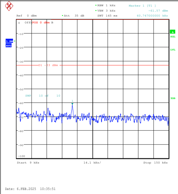
Band26(824-849)-3MHz-QPSK-27025-15RB#0-0. 009~0.15-PASS
