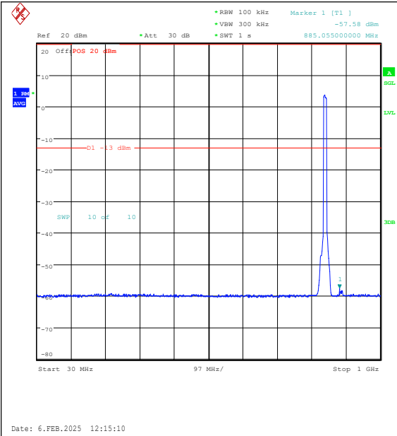
Band26(824-849)-10MHz-QPSK-26990-50RB#0-3 0~1000-PASS
