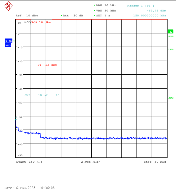
Band26(824-849)-3MHz-QPSK-27025-15RB#0-0. 15~30-PASS
