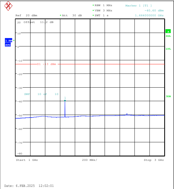
Band26(824-849)-10MHz-QPSK-26915-1RB#0-10 00~3000-PASS
