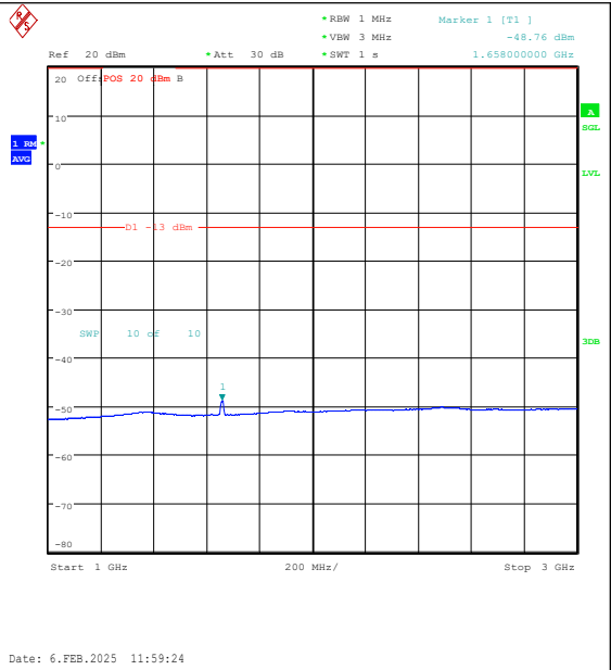
Band26(824-849)-10MHz-QPSK-26840-50RB#0-1 000~3000-PASS
