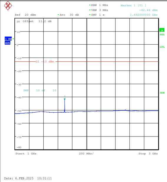
Band26(824-849)-3MHz-QPSK-27025-1RB#0-100 0~3000-PASS
