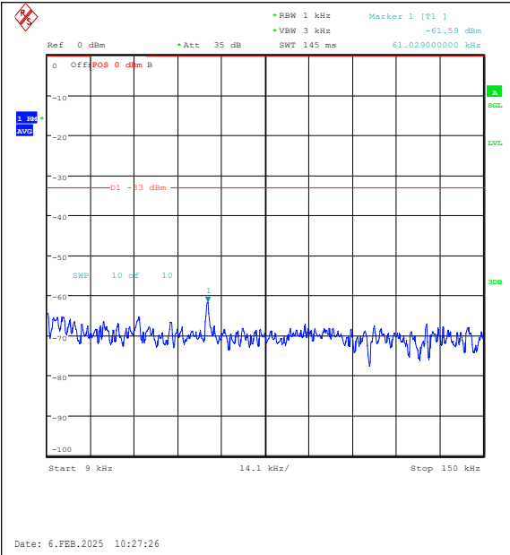
Band26(824-849)-3MHz-QPSK-26915-15RB#0-0. 009~0.15-PASS
