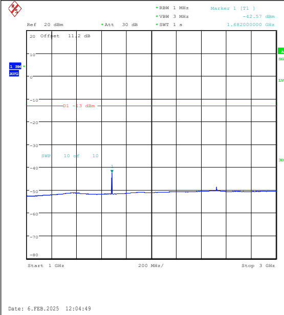
Band26(824-849)-10MHz-QPSK-26915-1RB#49-1 000~3000-PASS
