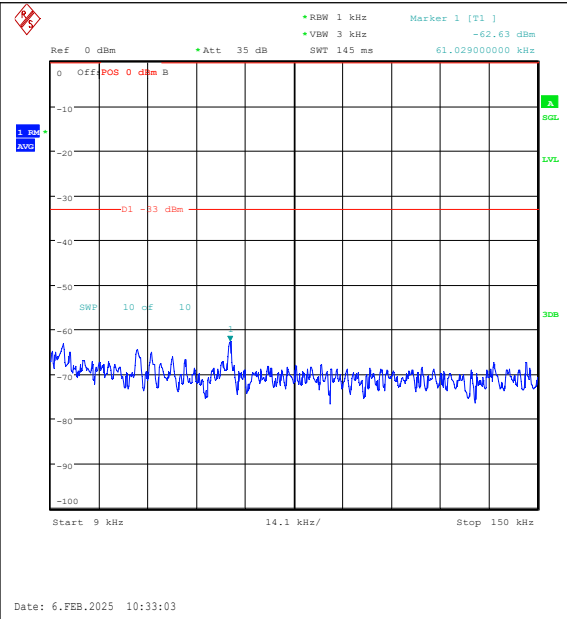
Band26(824-849)-3MHz-QPSK-27025-1RB#14-0. 009~0.15-PASS
