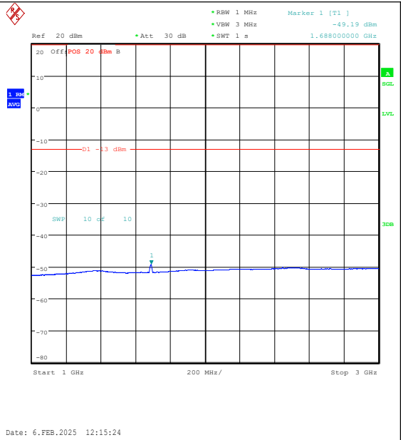
Band26(824-849)-10MHz-QPSK-26990-50RB#0-1 000~3000-PASS
