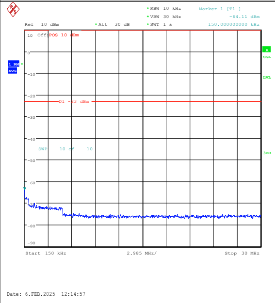
Band26(824-849)-10MHz-QPSK-26990-50RB#0-0 .15~30-PASS
