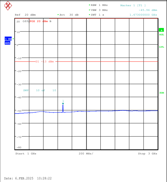
Band26(824-849)-3MHz-QPSK-26915-15RB#0-10 00~3000-PASS
