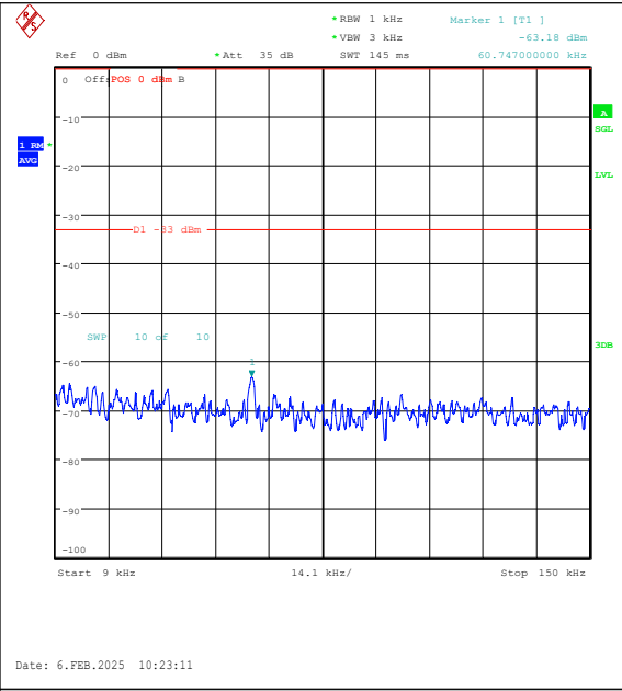
Band26(824-849)-3MHz-16QAM-26915-1RB#0-0. 009~0.15-PASS
