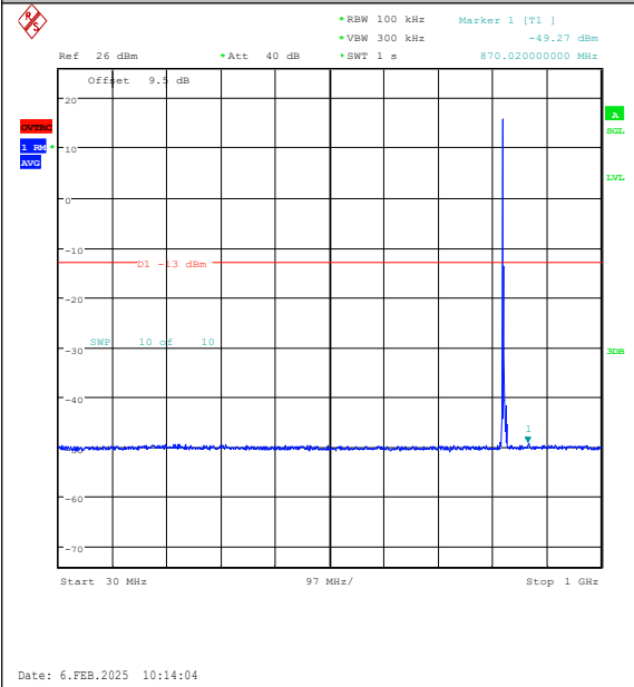
Band26(824-849)-3MHz-QPSK-26805-1RB#0-30~ 1000-PASS
