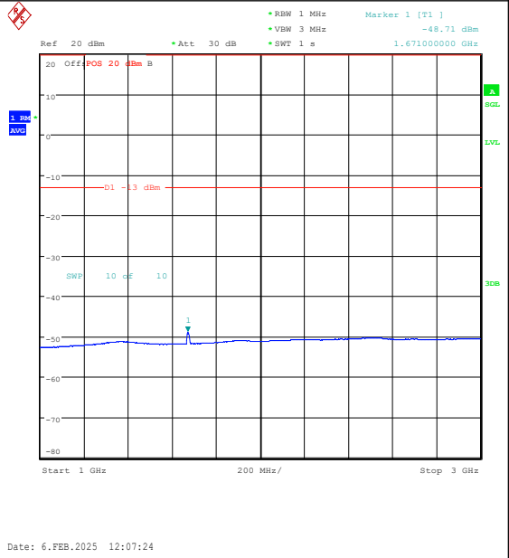
Band26(824-849)-10MHz-QPSK-26915-50RB#0-1 000~3000-PASS
