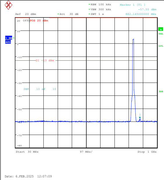
Band26(824-849)-10MHz-QPSK-26915-50RB#0-3 0~1000-PASS
