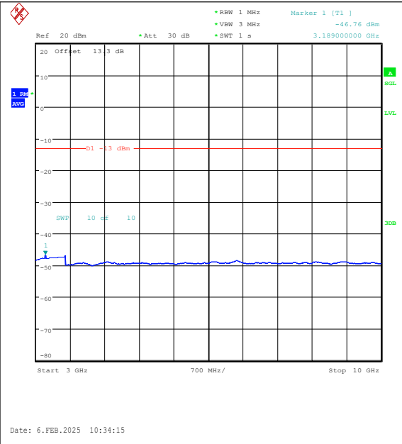
Band26(824-849)-3MHz-QPSK-27025-1RB#14-30 00~10000-PASS
