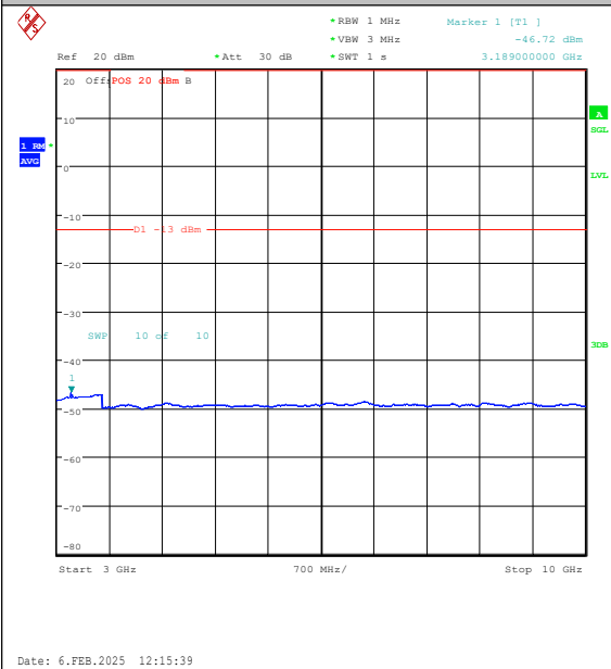
Band26(824-849)-10MHz-QPSK-26990-50RB#0-3 000~10000-PASS
