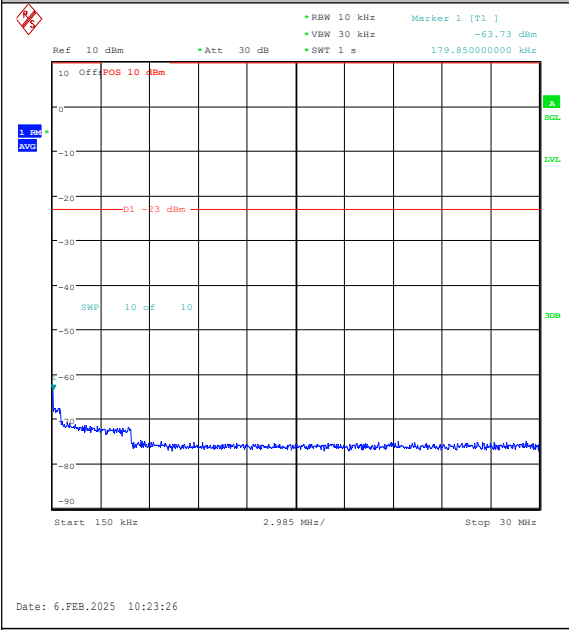
Band26(824-849)-3MHz-16QAM-26915-1RB#0-0. 15~30-PASS
