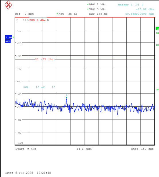
Band26(824-849)-3MHz-QPSK-26915-1RB#0-0.0 09~0.15-PASS
