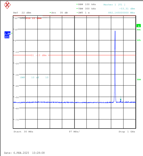
Band26(824-849)-3MHz-QPSK-26915-15RB#0-30 ~1000-PASS
