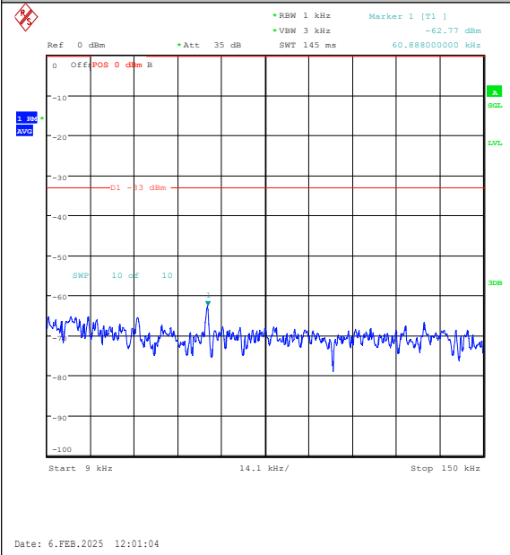
Band26(824-849)-10MHz-QPSK-26915-1RB#0-0.009~0.15-PASS
