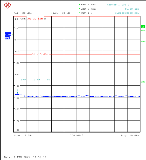
Band26(824-849)-10MHz-QPSK-26840-50RB#0-3 000~10000-PASS
