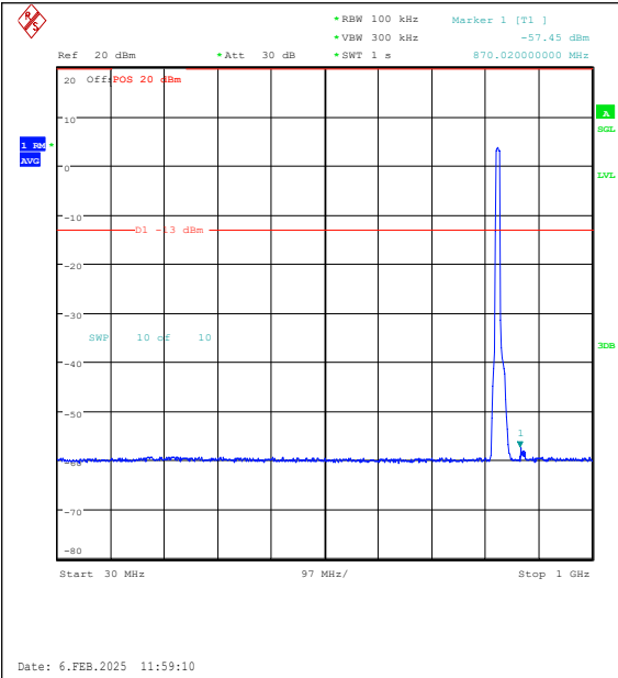
Band26(824-849)-10MHz-QPSK-26840-50RB#0-3 0~1000-PASS
