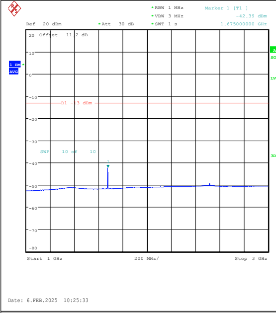
Band26(824-849)-3MHz-QPSK-26915-1RB#14-10 00~3000-PASS
