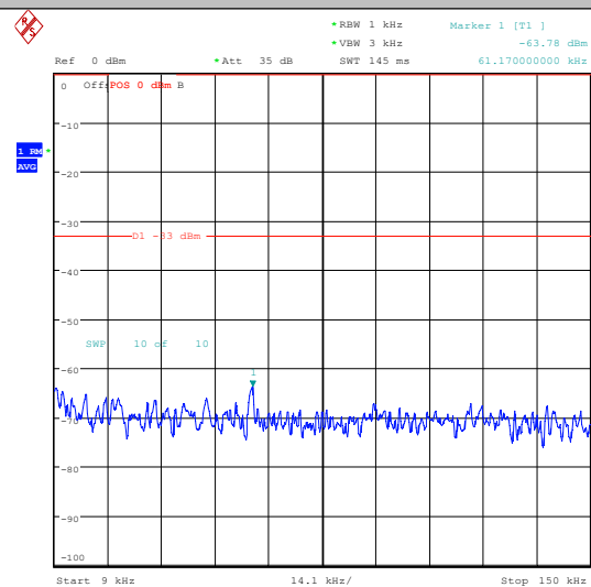
Band26(824-849)-3MHz-QPSK-26805-1RB#14-10 00~3000-PASS
