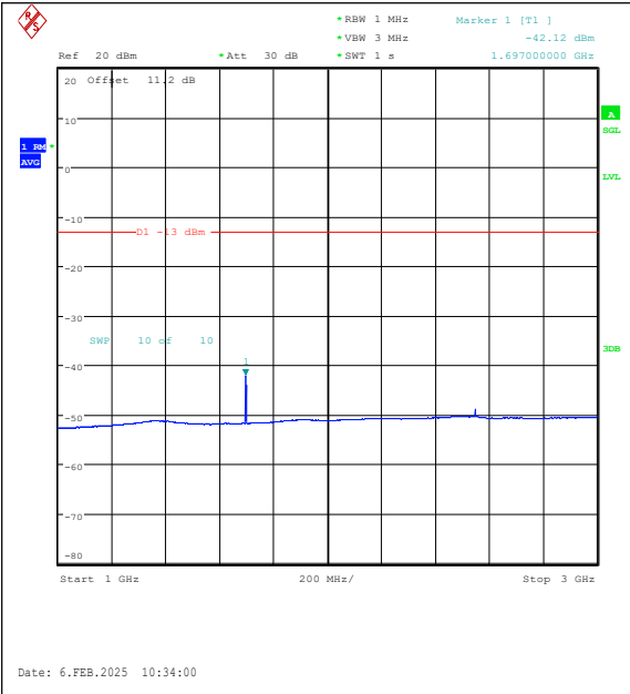
Band26(824-849)-3MHz-QPSK-27025-1RB#14-10 00~3000-PASS
