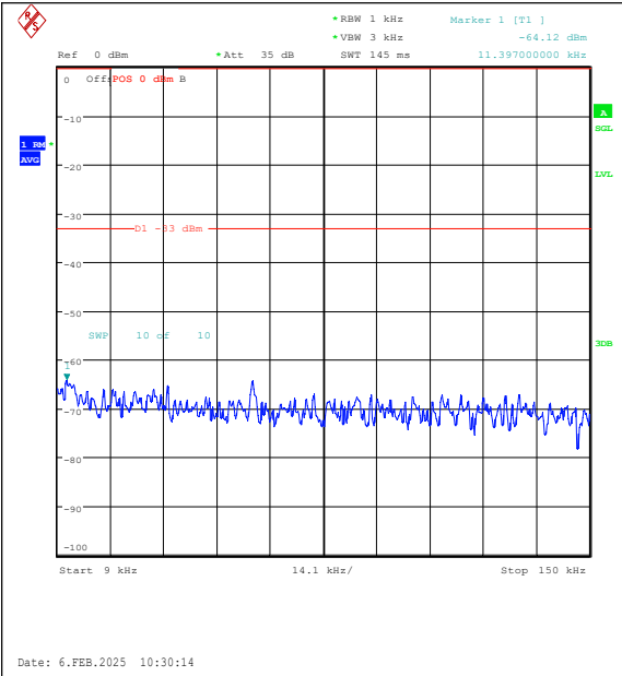
Band26(824-849)-3MHz-QPSK-27025-1RB#0-0.0 09~0.15-PASS
