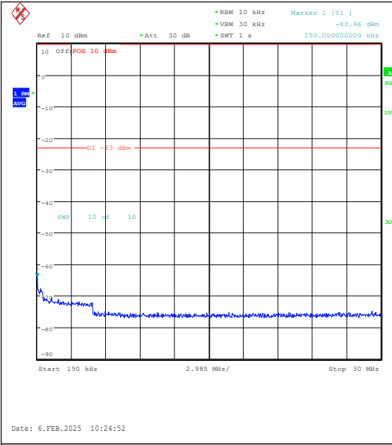
Band26(824-849)-3MHz-QPSK-26915-1RB#14-0. 15~30-PASS
