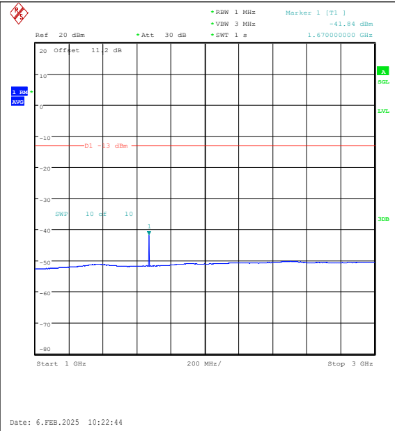
Band26(824-849)-3MHz-QPSK-26915-1RB#0-1000~3000-PASS
