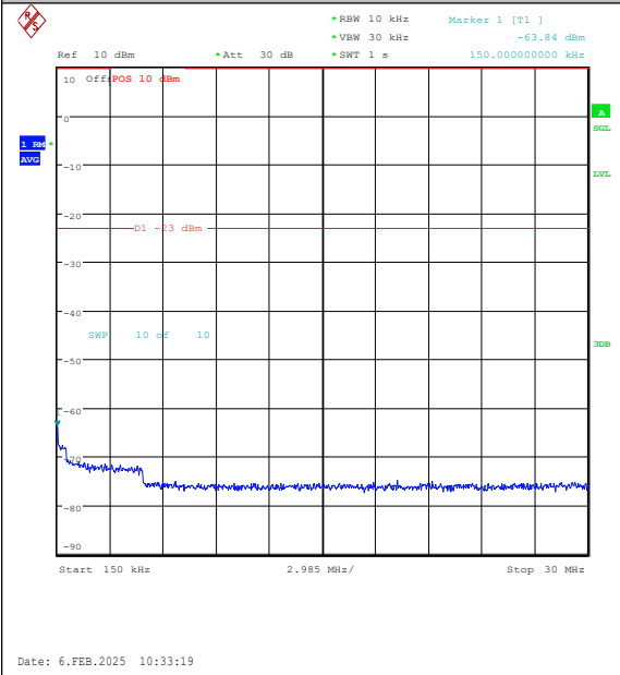
Band26(824-849)-3MHz-QPSK-27025-1RB#14-0. 15~30-PASS
