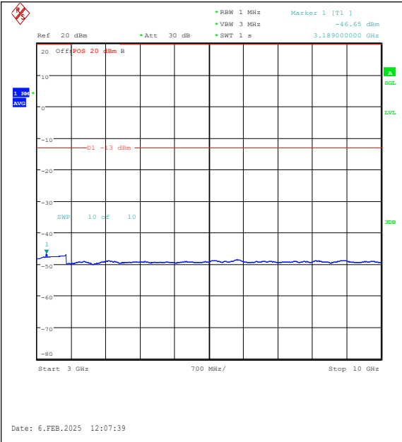
Band26(824-849)-10MHz-QPSK-26915-50RB#0-3 000~10000-PASS
