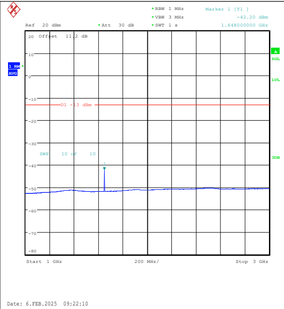
Band26(824-849)-1.4MHz-QPSK-26797-1RB#0-1 000~3000-PASS
