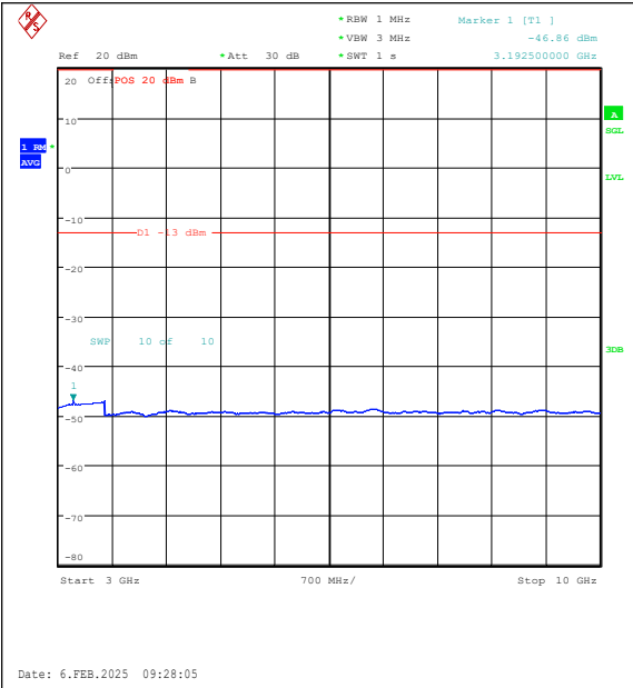
Band26(824-849)-1.4MHz-QPSK-26797-6RB#0-3 000~10000-PASS
