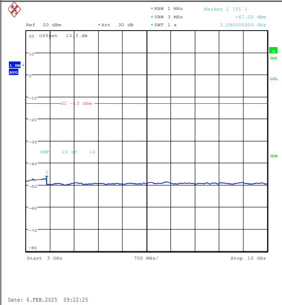
Band26(824-849)-1.4MHz-QPSK-26797-1RB#0-3 000~10000-PASS
