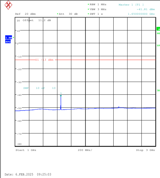
Band26(824-849)-1.4MHz-QPSK-26797-1RB#5-1 000~3000-PASS
