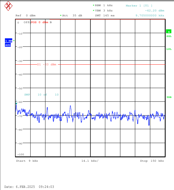
Band26(824-849)-1.4MHz-QPSK-26797-1RB#5-0. 009~0.15-PASS
