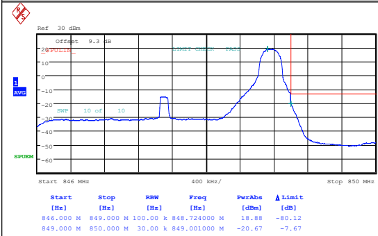
Band26(824-849)-3MHz-QPSK-27025-15RB#0-P ASS
