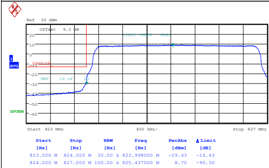
Band26(824-849)-3MHz-QPSK-26805-1RB#0-PA SS
