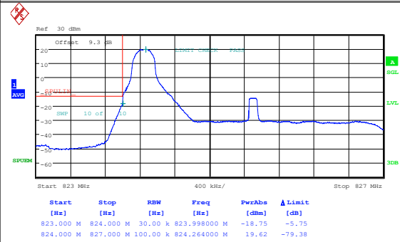
Band26(824-849)-3MHz-QPSK-26805-1RB#14-P ASS
