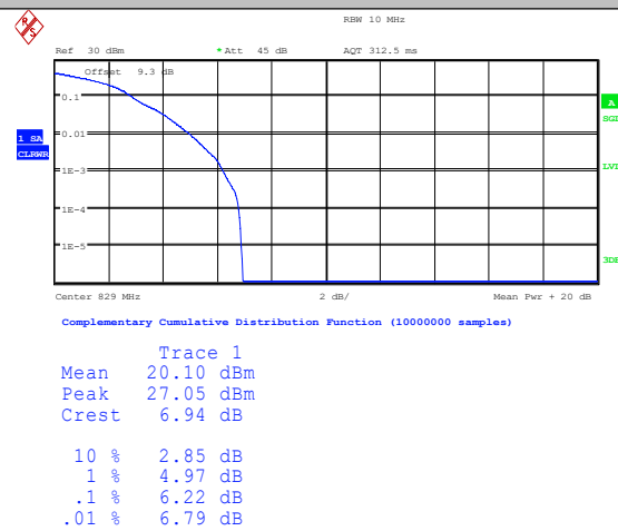
Band26(824-849)-10MHz-QPSK-26840-1RB#0-P ASS
