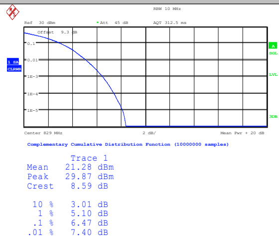
Band26(824-849)-10MHz-QPSK-26840-50RB#0-P ASS
