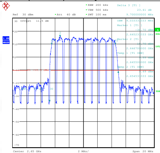
Band41(2535-2655)-10MHz-QPSK-40590-50RB#0-PASS
