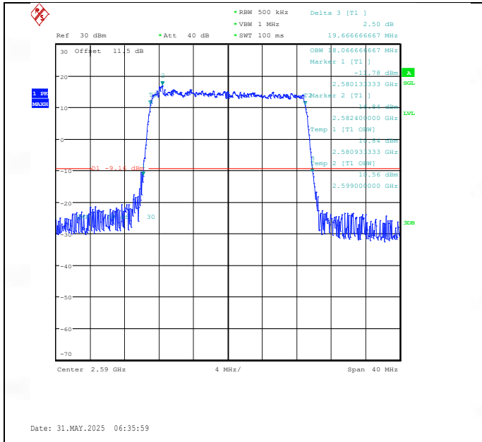
Band41(2535-2655)-20MHz-QPSK-40590-100RB#0-PASS
