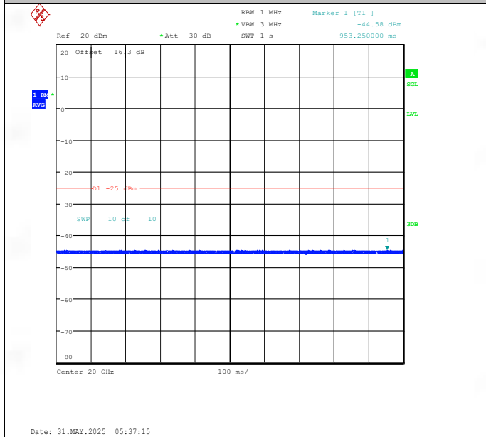
Band41(2535-2655)-10MHz-QPSK-40090-1RB#0-20000~27000-PASS
