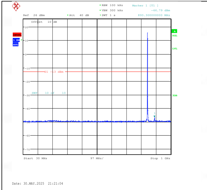
Band26(824-849)-3MHz-QPSK-27025-1RB#0-30~1000-PASS
