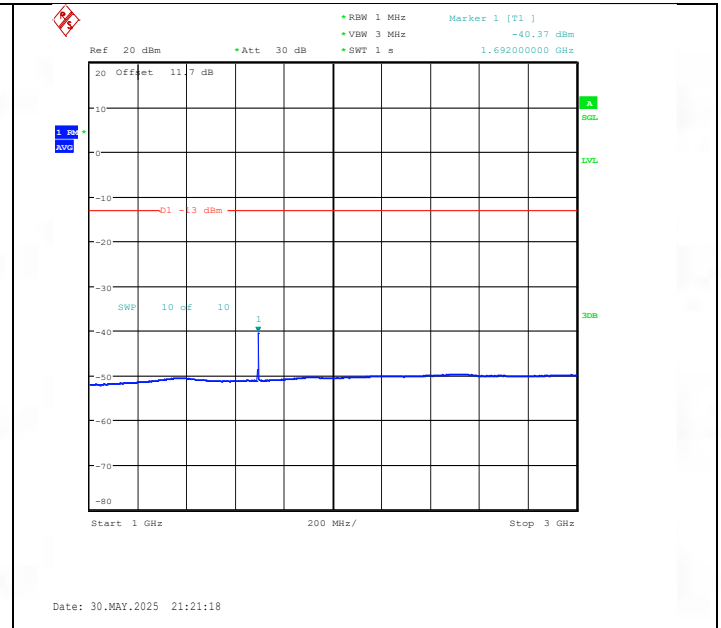
Band26(824-849)-3MHz-QPSK-27025-1RB#0-1000~3000-PASS
