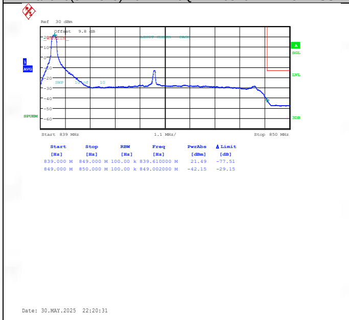
Band26(824-849)-10MHz-QPSK-26990-1RB#0-PASS
