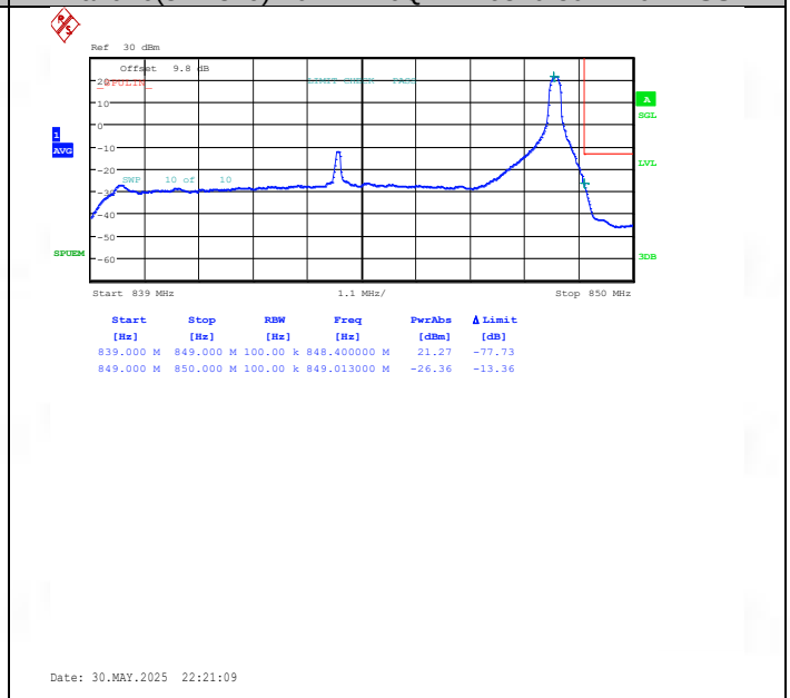
Band26(824-849)-10MHz-QPSK-26990-1RB#49-PASS
