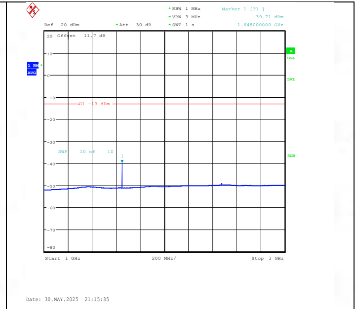
Band26(824-849)-3MHz-QPSK-26805-1RB#0-1000~3000-PASS
