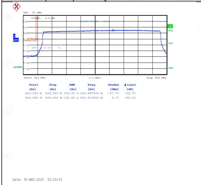
Band26(824-849)-10MHz-QPSK-26840-50RB#0-PASS
