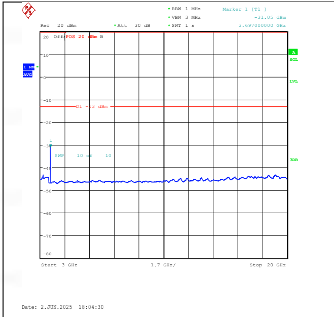
Band25-15MHz-QPSK-26115-1RB#0-3000~20000-PASS
