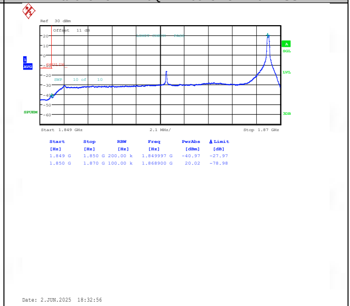
Band25-20MHz-QPSK-26140-1RB#99-PASS
