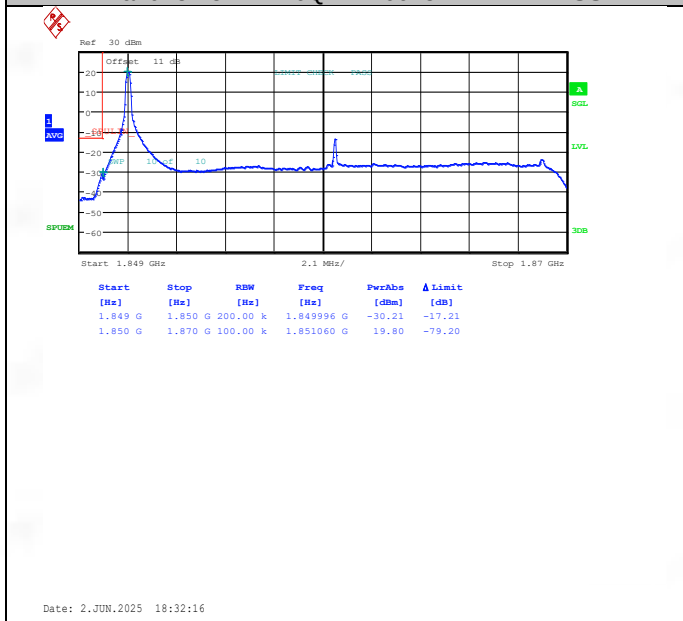
Band25-20MHz-QPSK-26140-1RB#0-PASS
