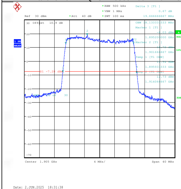
Band25-20MHz-QPSK-26590-100RB#0-PASS
