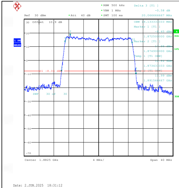
Band25-20MHz-QPSK-26365-100RB#0-PASS
