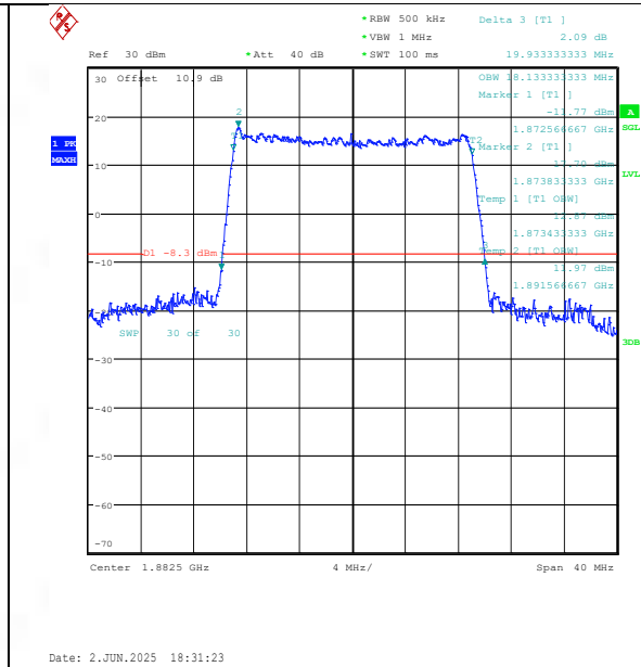
Band25-20MHz-16QAM-26365-100RB#0-PASS
