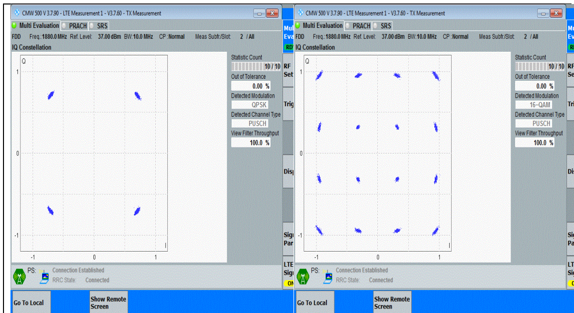
Band2-10MHz-QPSK-18900-50RB#0-PASS
