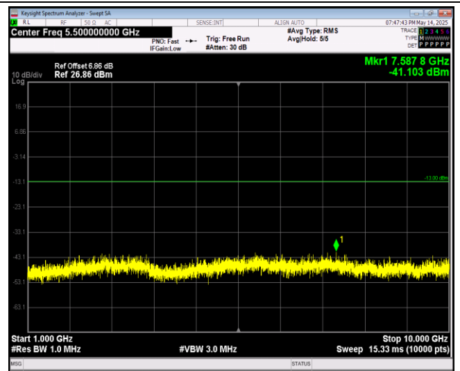
Band5-1.4MHz-QPSK-20525-1RB#0-Range2:1000~1 0000MHz
