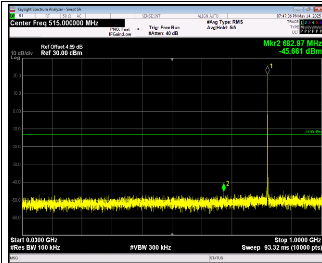
Band5-1.4MHz-QPSK-20525-1RB#0-Range1:30~100 0MHz
