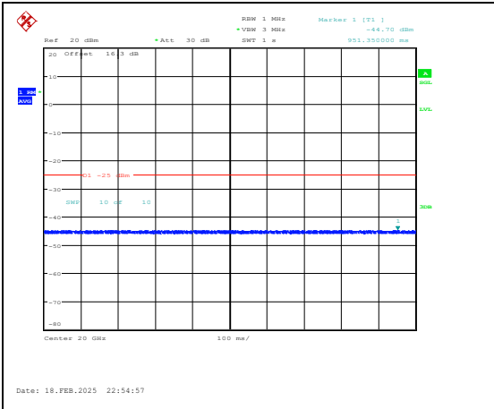
Band38-15MHz-QPSK-38175-1RB#0-20000~270 00-PASS
