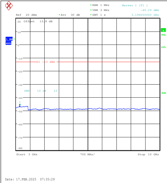
Band26(824-849)-1.4MHz-QPSK-26797-1RB#0-3 000~10000-PASS
