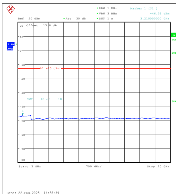
Band26(824-849)-10MHz-QPSK-26915-1RB#0-3 000~10000-PASS
