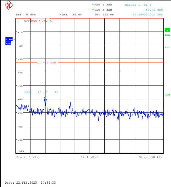
Band26(824-849)-10MHz-QPSK-26840-1RB#0-0. 009~0.15-PASS
