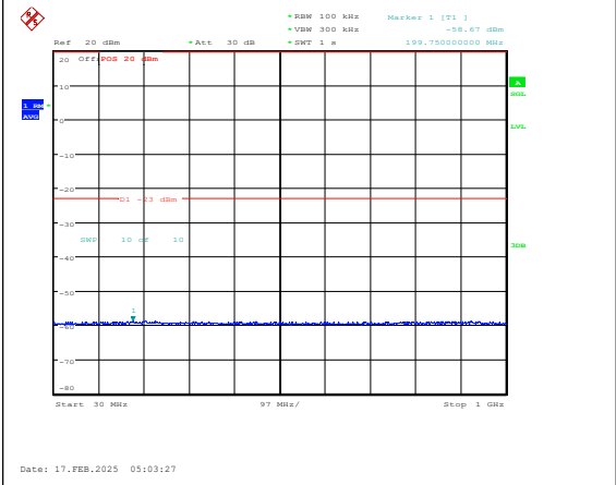
Band25-20MHz-QPSK-26140-1RB#0-30~1000-P ASS
