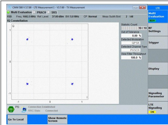
Band25-5MHz-QPSK-26365-25RB#0-PASS
