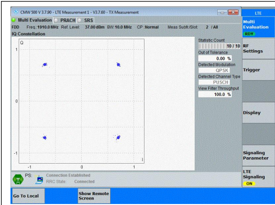
Band25-10MHz-QPSK-26640-50RB#0-PASS
