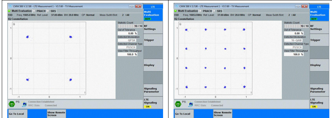
Band25-20MHz-QPSK-26590-100RB#0-PASS
