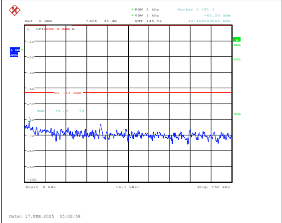
Band25-20MHz-QPSK-26140-1RB#0-0.009~0.15 -PASS
