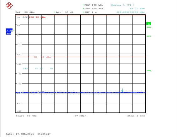
Band25-20MHz-QPSK-26365-1RB#0-30~1000-P ASS
