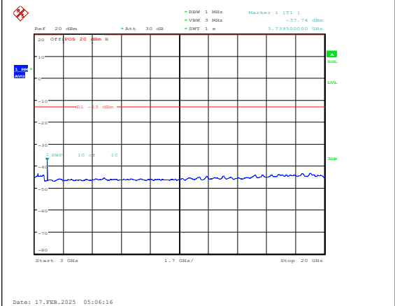
Band25-20MHz-QPSK-26365-1RB#0-3000~2000 0-PASS
