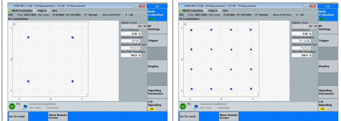
Band25-20MHz-QPSK-26365-100RB#0-PASS
