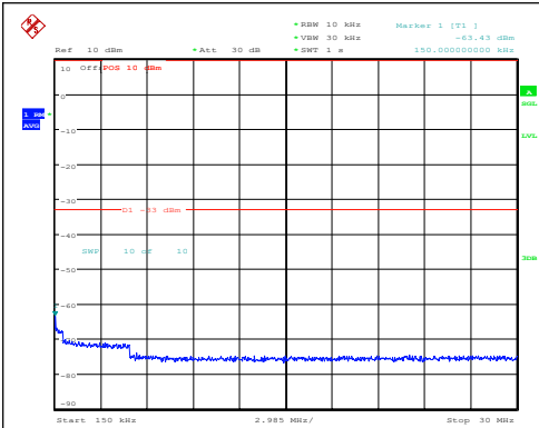
Band25-20MHz-16QAM-26365-1RB#0-0.15~30-P ASS
