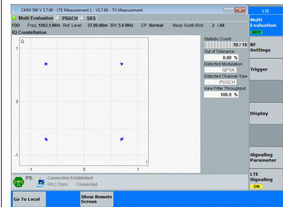
Band25-3MHz-QPSK-26365-15RB#0-PASS
