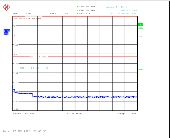
Band25-20MHz-QPSK-26365-1RB#0-0.15~30-PA SS
