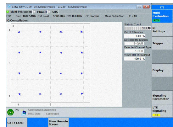
Band25-10MHz-16QAM-26365-50RB#0-PASS
