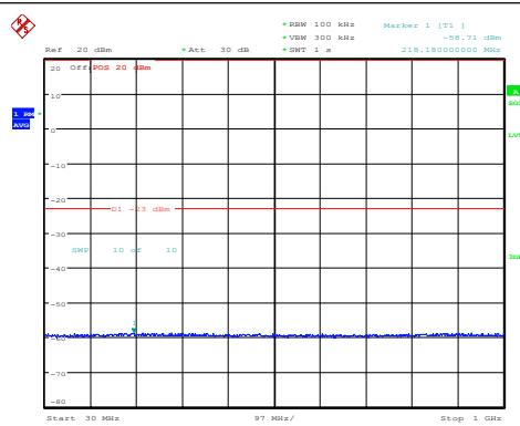
Band25-20MHz-16QAM-26365-1RB#0-30~1000-P ASS
