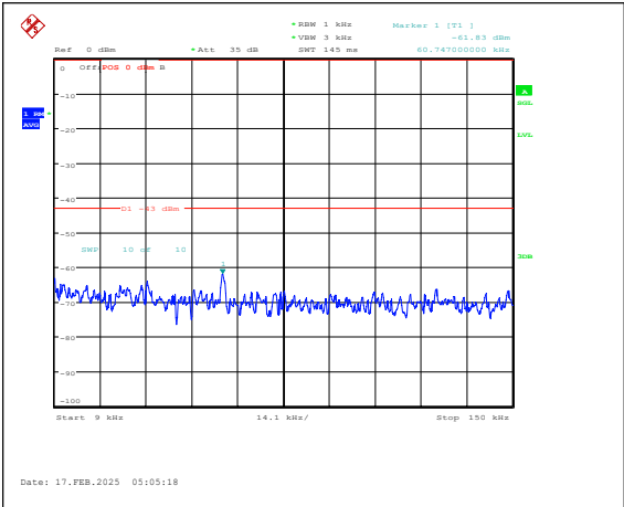
Band25-20MHz-QPSK-26365-1RB#0-0.009~0.15 -PASS
