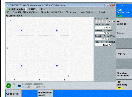
Band25-10MHz-QPSK-26365-50RB#0-PASS
