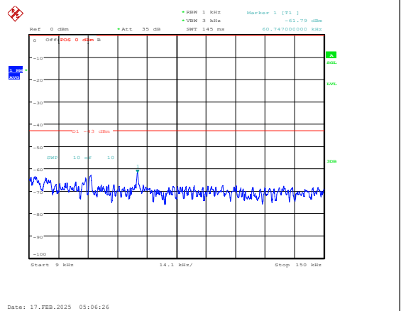
Band25-20MHz-16QAM-26365-1RB#0-0.009~0.15 -PASS
