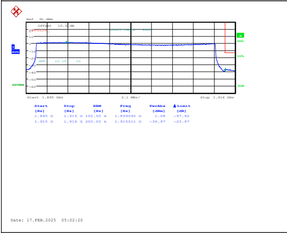
Band25-20MHz-QPSK-26590-100RB#0-PASS
