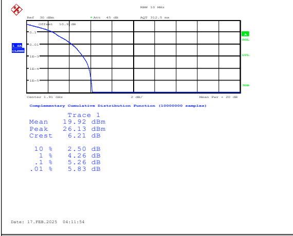
Band25-10MHz-QPSK-26640-1RB#0-PASS
