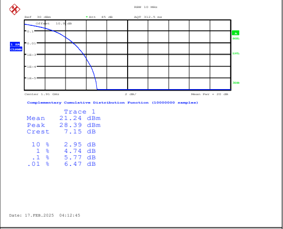
Band25-10MHz-QPSK-26640-50RB#0-PASS
