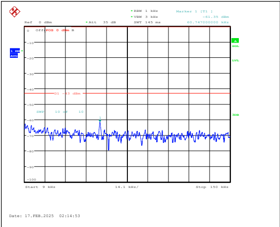
Band25-1.4MHz-QPSK-26365-1RB#0-0.009~0.15 -PASS
