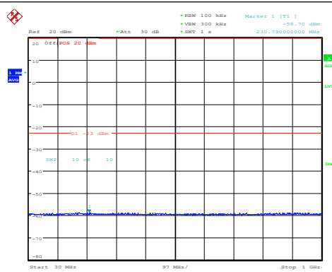
Band25-10MHz-16QAM-26365-1RB#0-30~1000-P ASS
