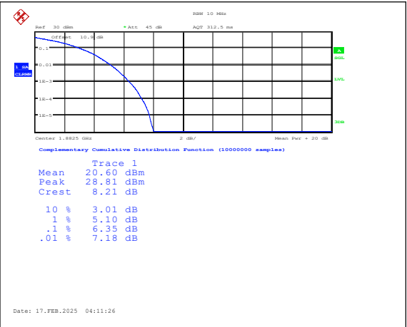
Band25-10MHz-16QAM-26365-50RB#0-PASS
