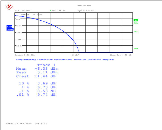
Band25-20MHz-QPSK-26140-1RB#0-PASS
