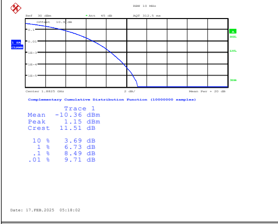
Band25-20MHz-QPSK-26365-1RB#0-PASS
