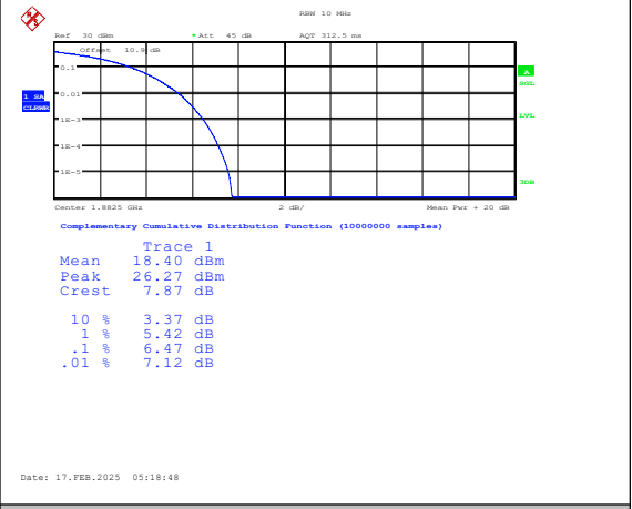
Band25-20MHz-QPSK-26365-100RB#0-PASS
