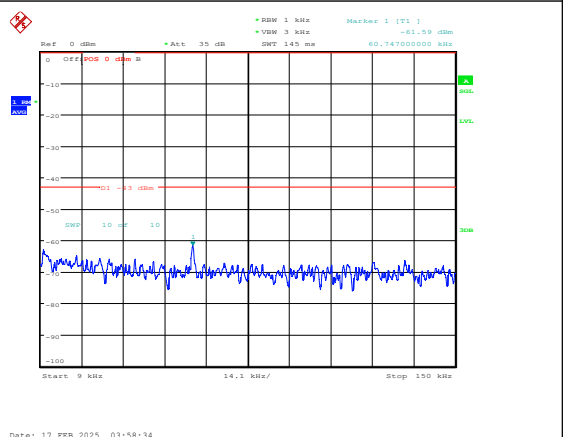
Band25-10MHz-16QAM-26365-1RB#0-0.009~0.15 -PASS
