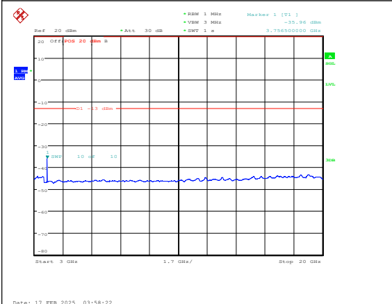
Band25-10MHz-QPSK-26365-1RB#0-3000~2000 0-PASS
