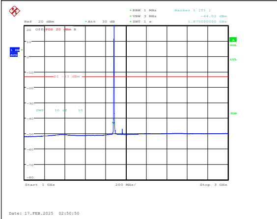
Band25-3MHz-16QAM-26365-1RB#0-1000~3000 -PASS
