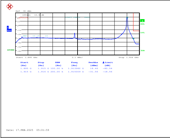
Band25-20MHz-16QAM-26590-1RB#99-PASS
