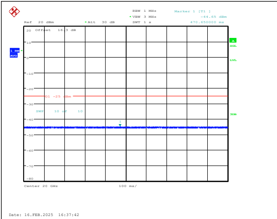
Band7-5MHz-QPSK-21425-1RB#0-20000~27000 -PASS
