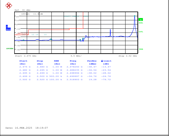
Band7-20MHz-QPSK-20850-1RB#99-PASS
