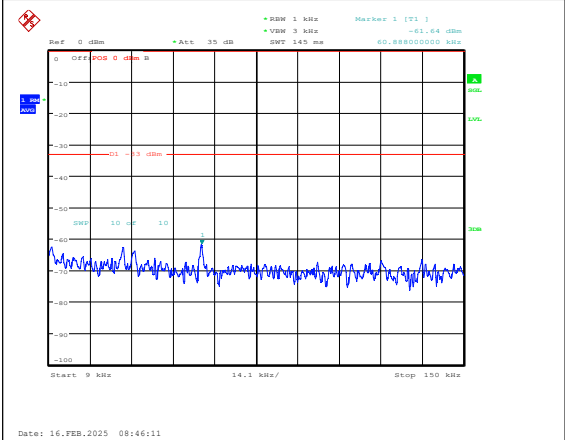
Band5-3MHz-QPSK-20635-1RB#0-0.009~0.15-PASS
