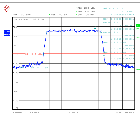
Band4-10MHz-QPSK-20000-50RB#0-PASS
