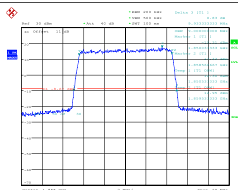
Band2-10MHz-QPSK-18650-50RB#0-PASS
