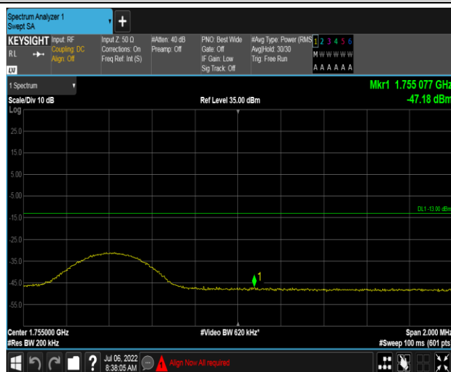
Band4-10MHz-QPSK-20350-1RB#0
