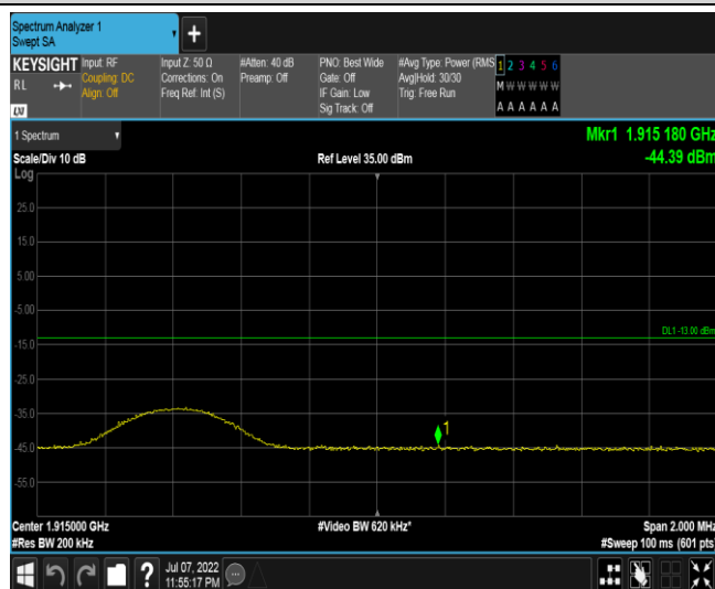
Band25-10MHz-QPSK-26640-1RB#0
