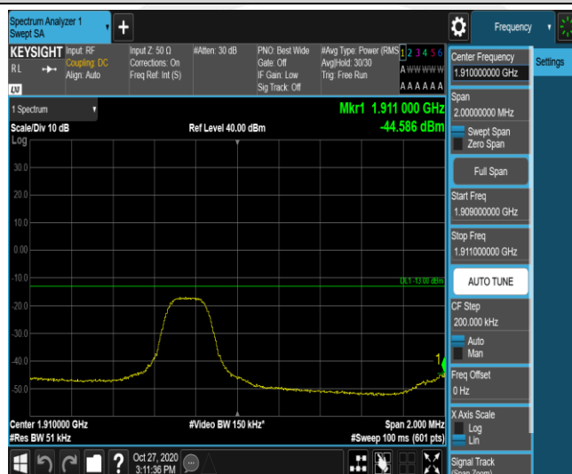
Band2-3MHz-QPSK-19185-1RB#14
