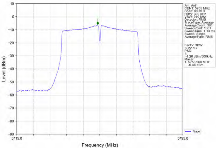
802.11ac(VHT40)_LCH_5755MHz_Ant1_NTNV
