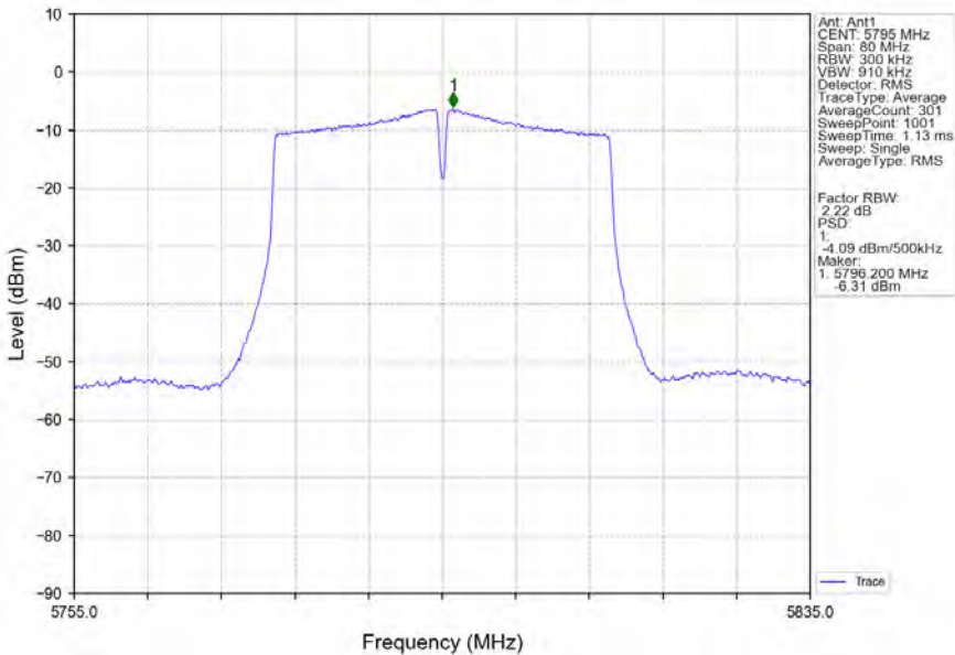
802.11n(HT40)_HCH_5795MHz_Ant1_NTNV
