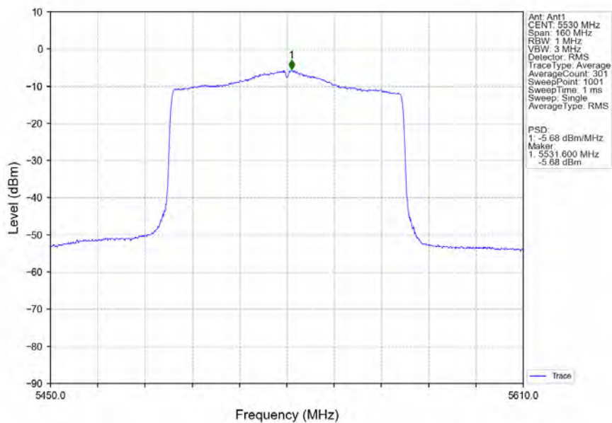
802.11ax(HEW80)_LCH_5530MHz_SU_ / _Ant1_NTNV
