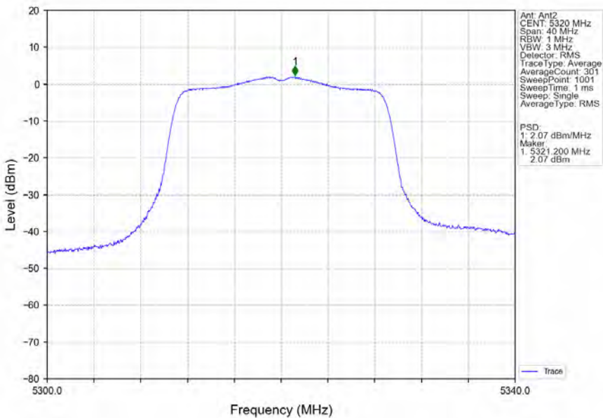
802.11n(HT20)_HCH_5320MHz_Ant2_NTNV
