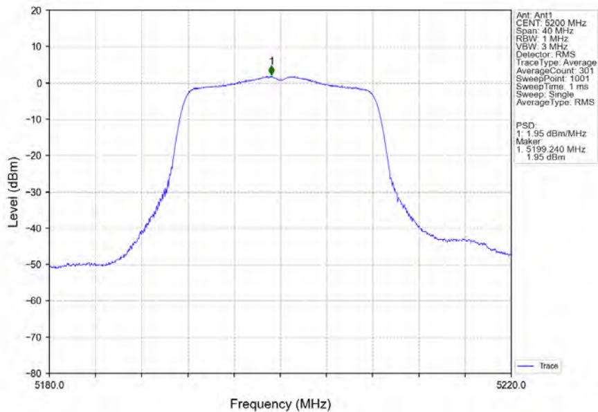
802.11a_MCH_5200MHz_Ant1_NTNV
