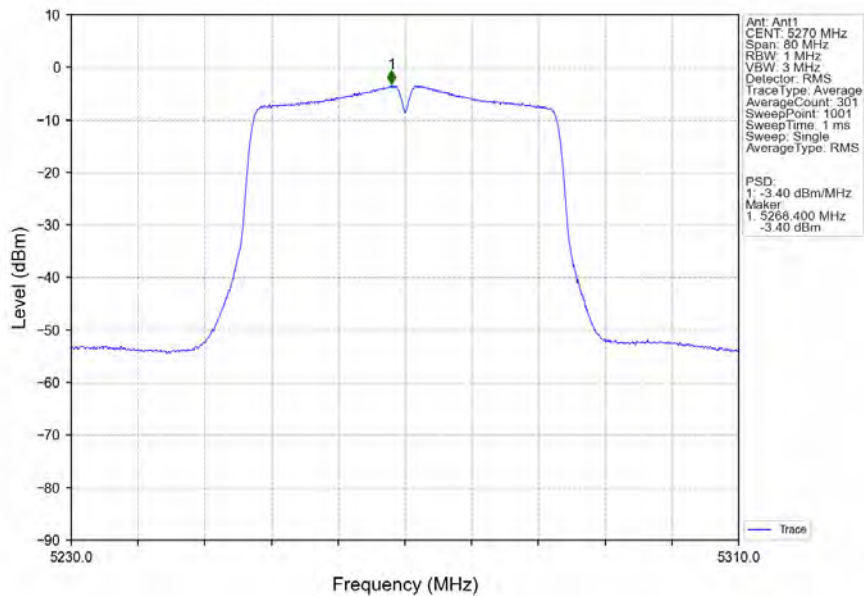
802.11ac(VHT40)_LCH_5270MHz_Ant1_NTNV
