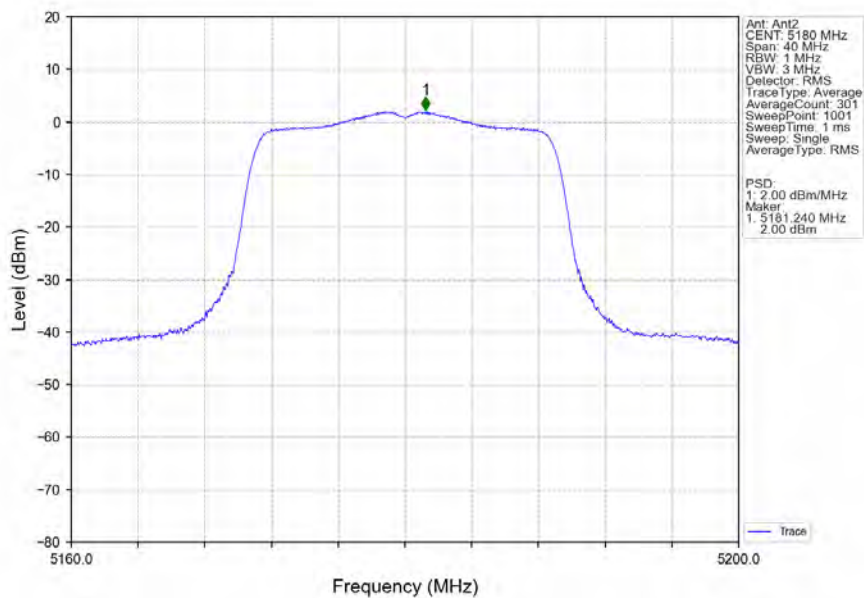
802.11n(HT20)_LCH_5180MHz_Ant2_NTNV
