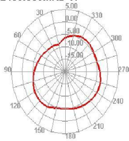
2450.000MHz H
