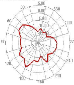
2450.000MHz E1
