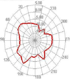
2400.000MHz E1
