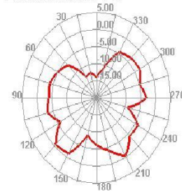
2500.000MHz E2
