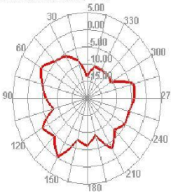
2500.000MHz E1
