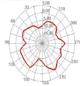
2400.000MHz E2
