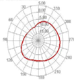
2400.000MHz H
