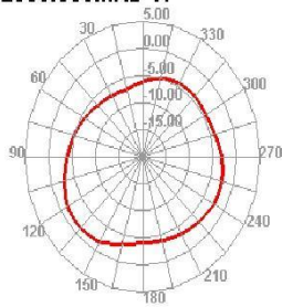
2500.000MHz H
