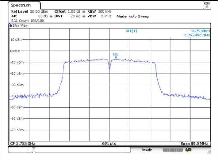
ANT 2
