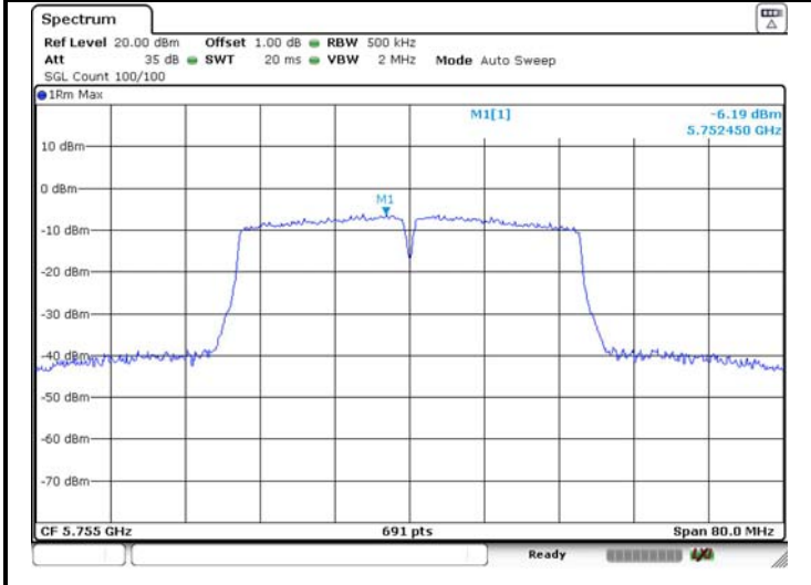
ANT 1
