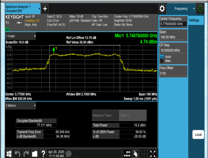
11AX80SISO-Ant1-5775
