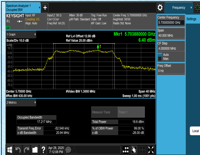
11A-Ant1-5700
