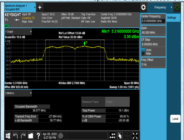
11N40SISO-Ant1-5310
