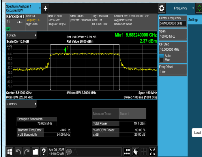
11AX80SISO-Ant1-5610
