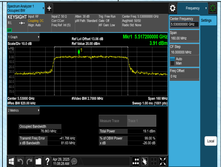
11AX80SISO-Ant1-5530
