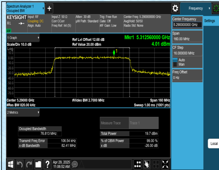
11AX80SISO-Ant1-5290
