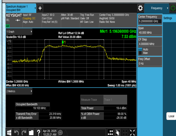
11AX20SISO-Ant1-5200
