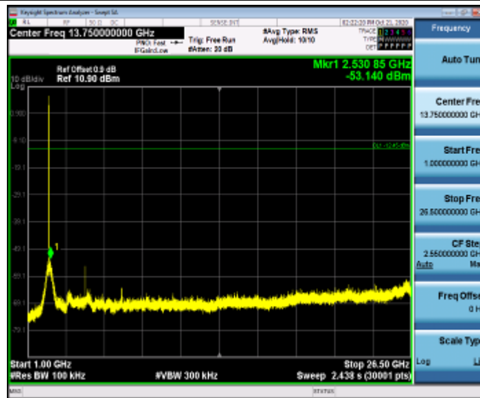
11B_Ant1_2442_0~Reference
