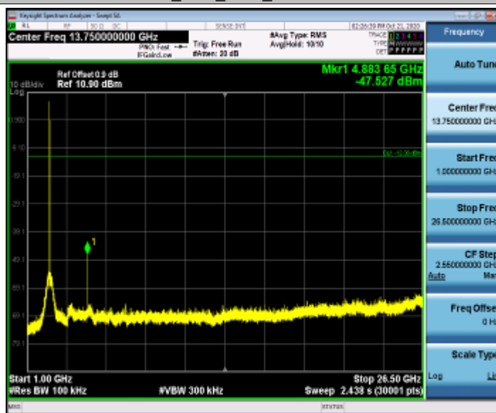
11B_Ant1_2442_1000~26500
