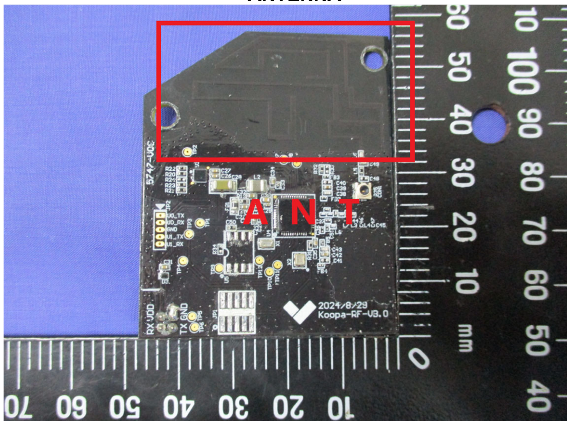
ANTENNA
