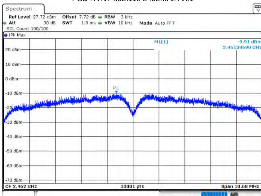
PSD NVNT 802.11b 2462MHz Ant1
