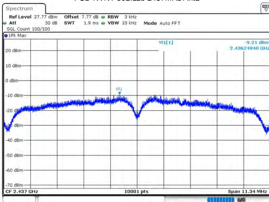
PSD NVNT 802.11b 2437MHz Ant1
