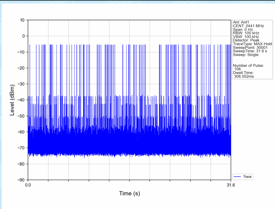
8DPSK_3DH5_HOPP_Ant1_NTNV
