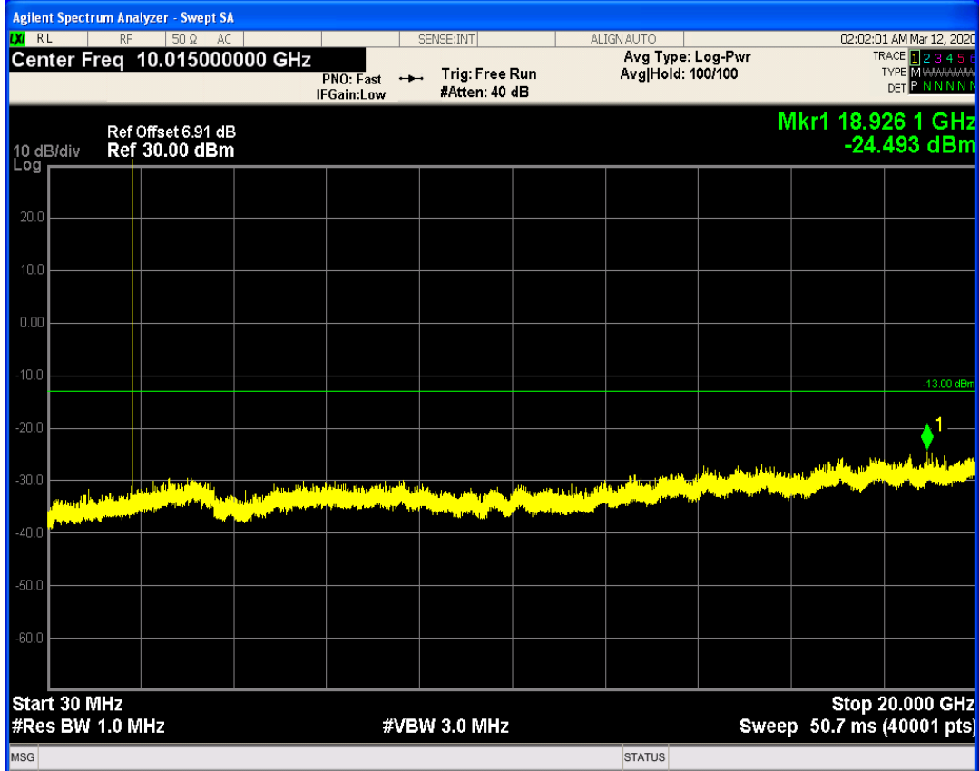
GPRS1900 Channel=810
