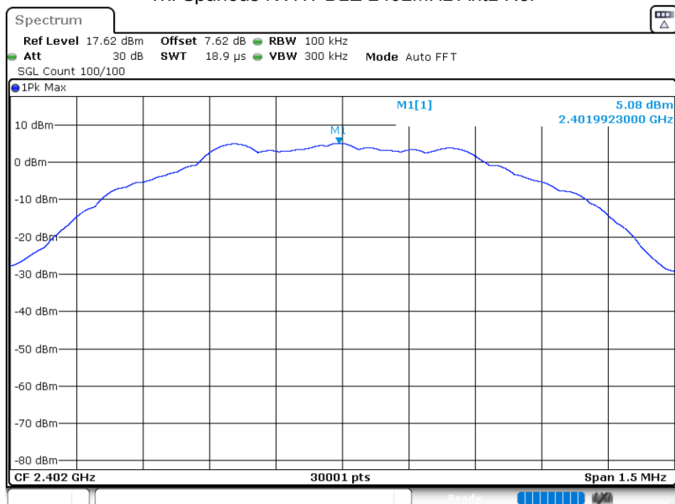
Tx. Spurious NVHT BLE 2402MHz Ant1 Ref
