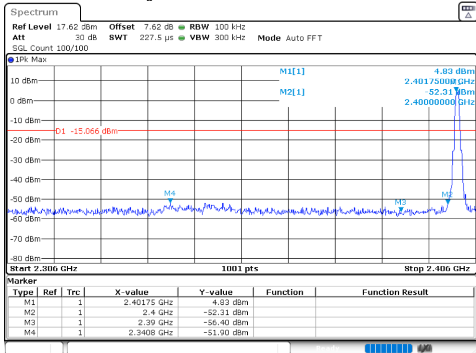
Band Edge NVHT BLE 2402MHz Ant1 Emission
