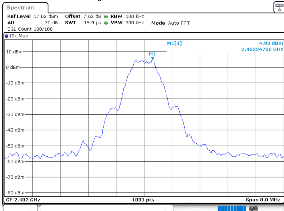
Band Edge NVHT BLE 2402MHz Ant1 Ref
