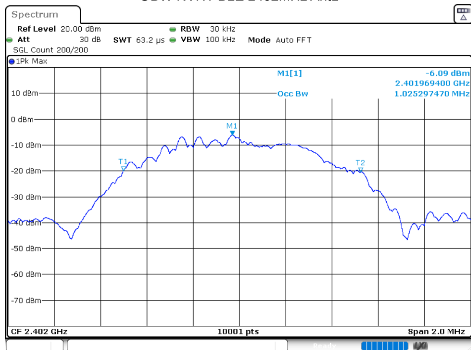
OBW NVHT BLE 2402MHz Ant1
