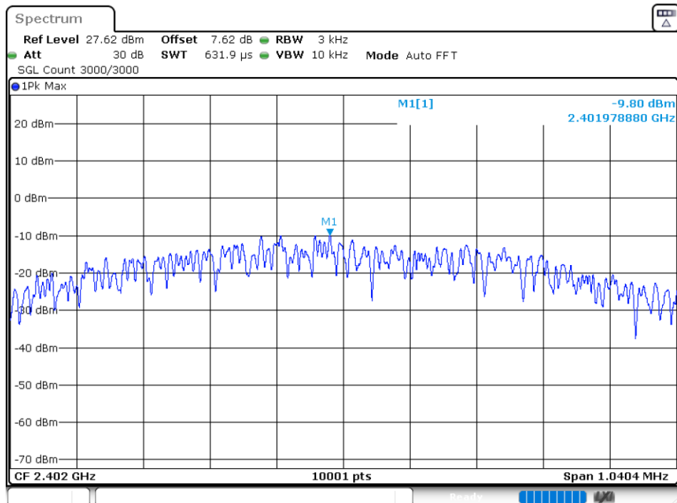
PSD NVHT BLE 2402MHz Ant1
