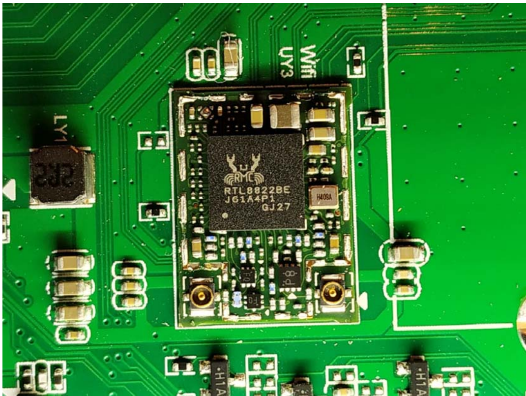
RF Module 2
