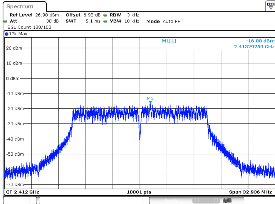
PSD 802.11g 2412MHz Ant1
