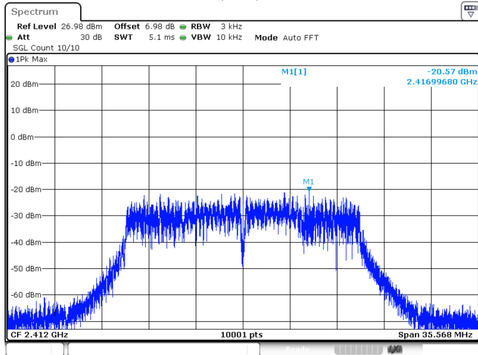
PSD 802.11n(HT20) 2412MHz Ant1
