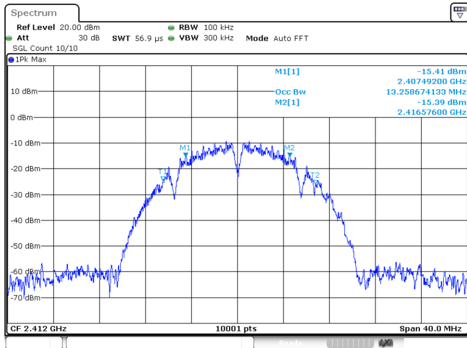
6dB BW 802.11b 2412MHz Ant1
