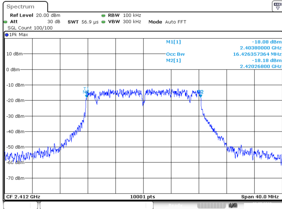
6dB BW 802.11g 2412MHz Ant1
