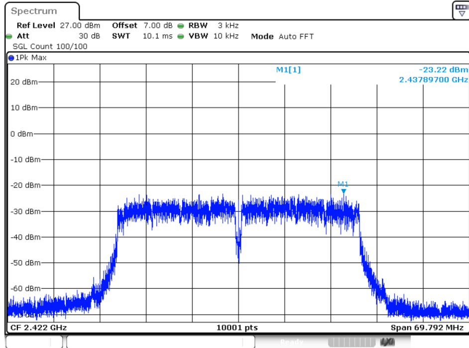
PSD 802.11n(HT40) 2422MHz Ant1
