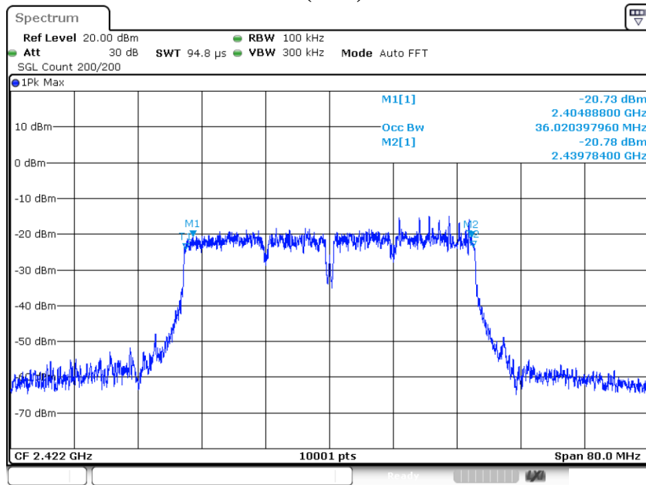
6dB BW 802.11n(HT40) 2422MHz Ant1
