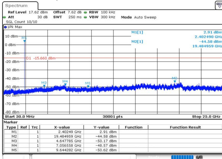
Tx. Spurious NVNT BLE 2402MHz Ant1 Emission
