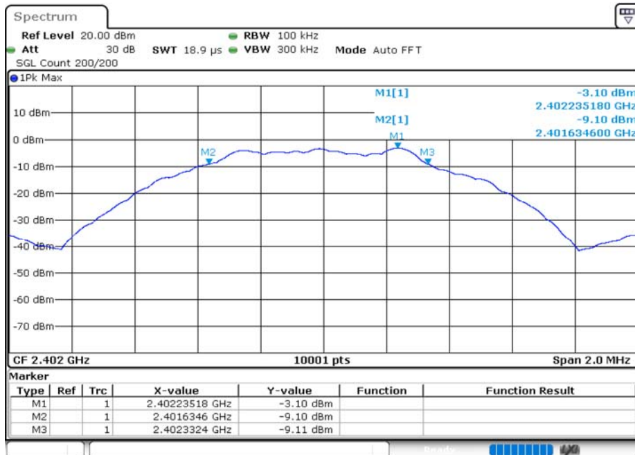
-6 dB BW NVNT BLE 2402MHz Ant1
