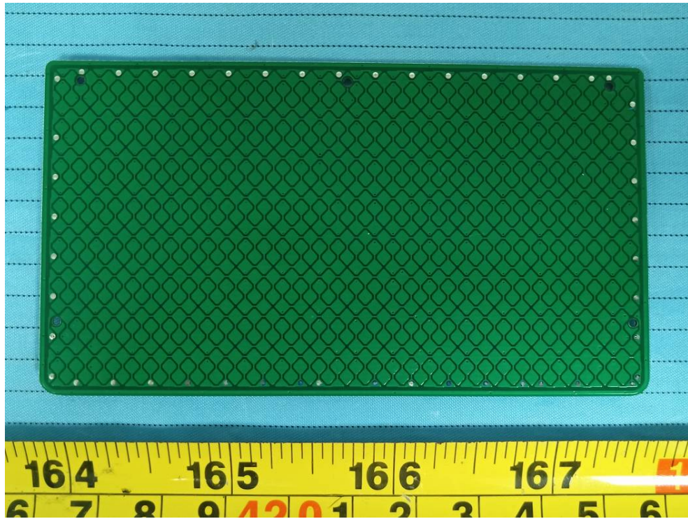
BT & Wi-FiAntenna
