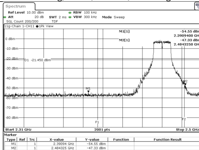
802.11g, CH11, Chain 1, Band edge
