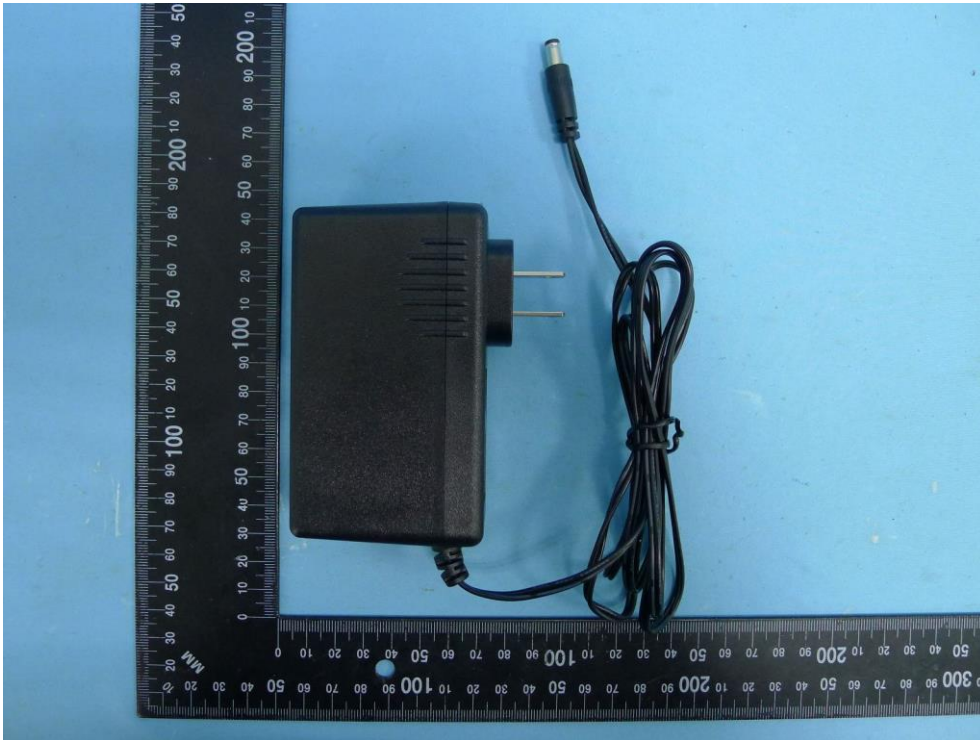
(13) EUT Photo
