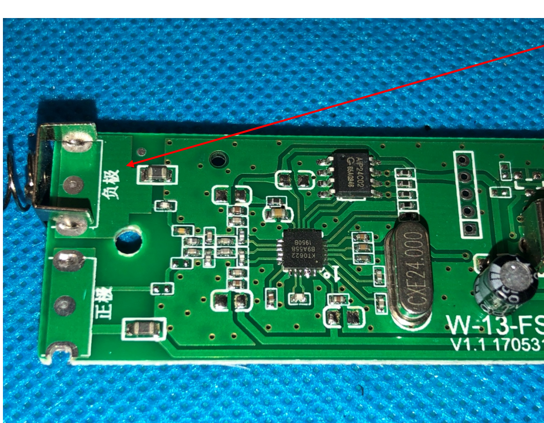
Antenna
