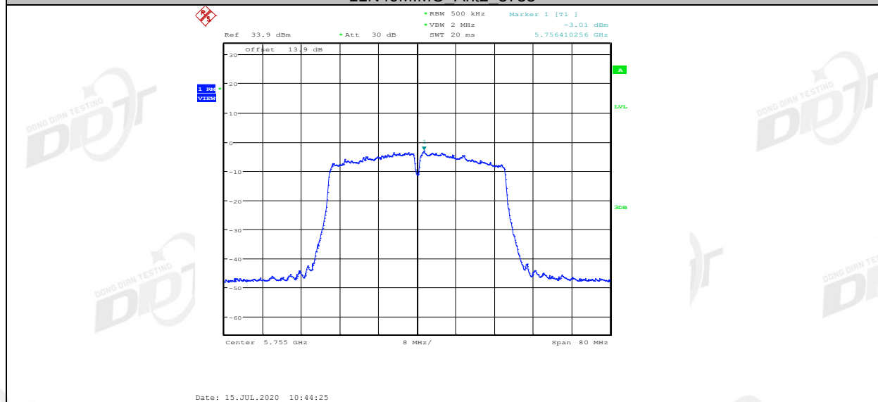
11N40MIMO_Ant3_5755
