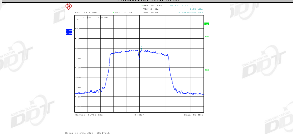
11N40MIMO_Ant4_5755
