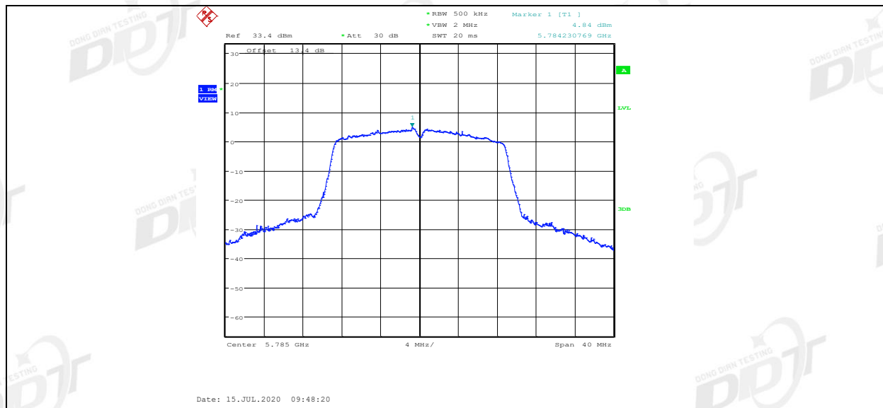
11N20MIMO_Ant3_5785
