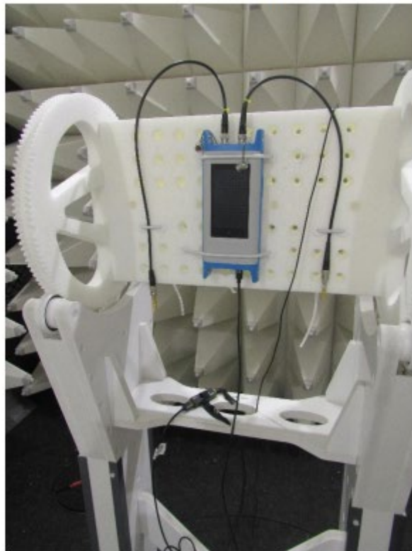
EUT Test Setup
