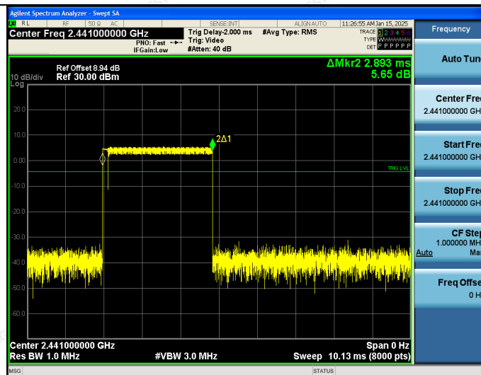
2-DH5
