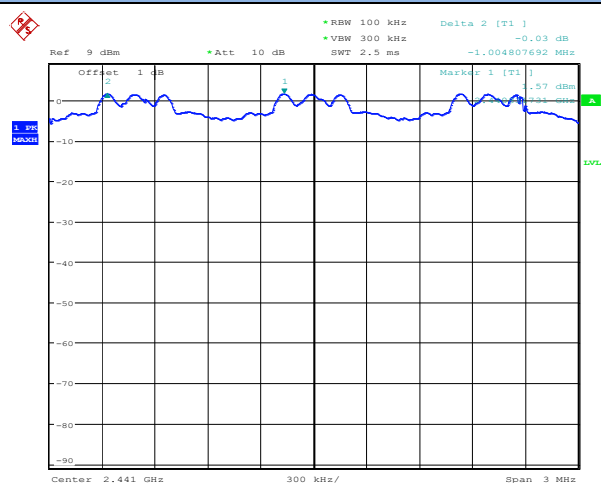
\pi/4 -DQPSK / Mid Channel
