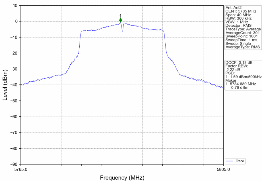
802.11a_MCH_5785MHz_Ant2_NTNV
