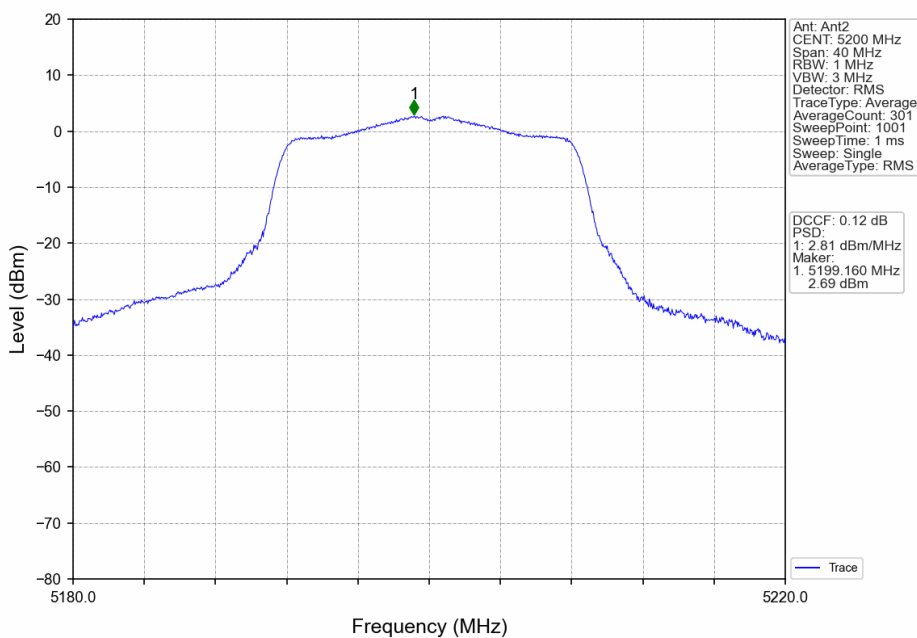
802.11a_MCH_5200MHz_Ant2_NTNV
