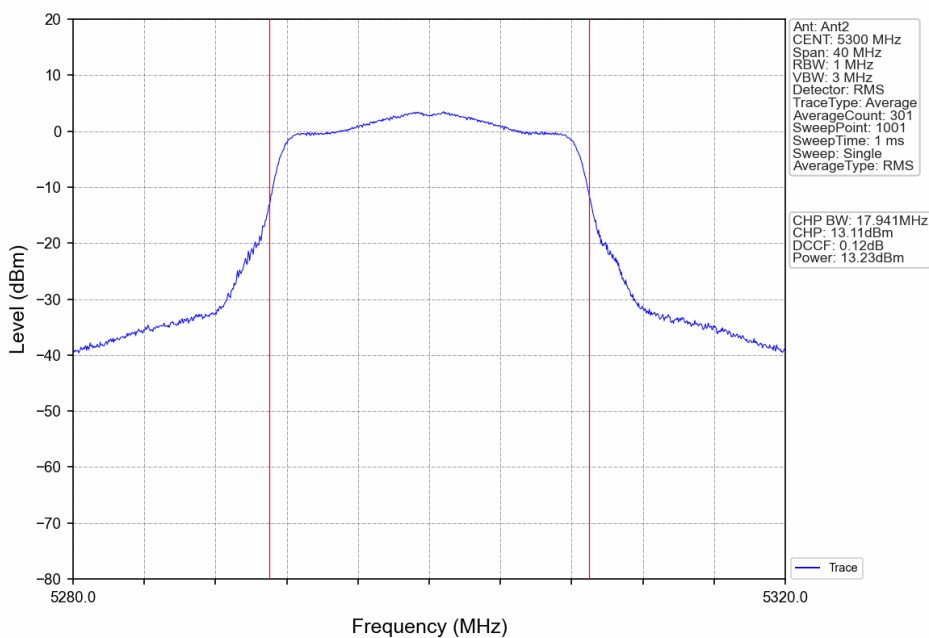
802.11a_MCH_5300MHz_Ant2_NTNV
