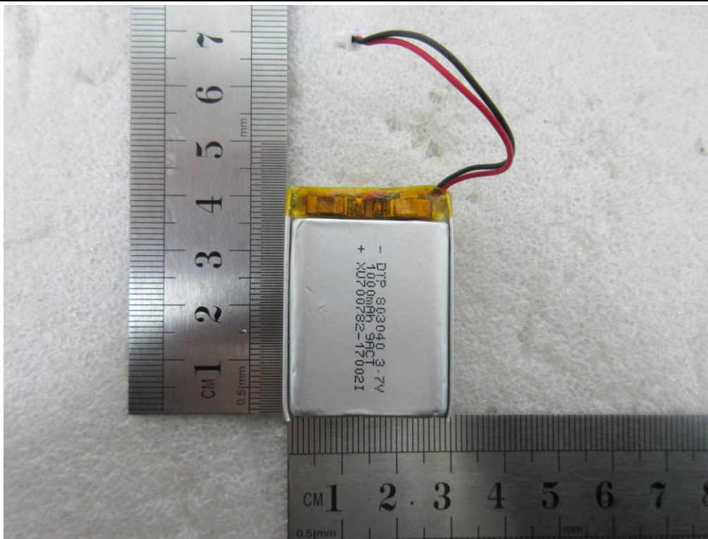
Battery_Front
