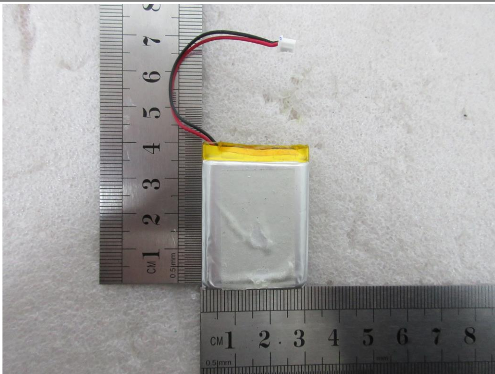
Battery_Rear
