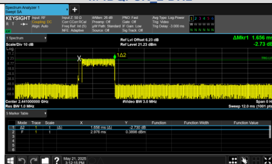
Pulse Width \pi/4 DQPSK 2-DH3
