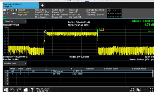
Pulse Width \pi/4 DQPSK 2-DH5
